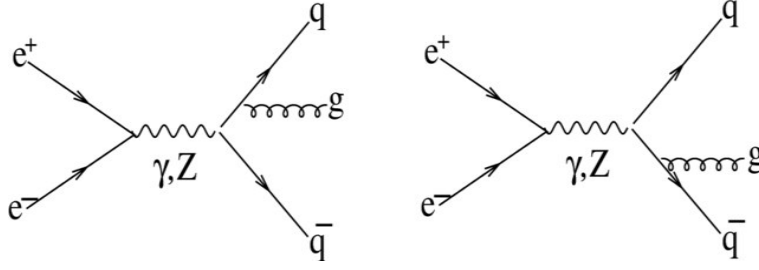
Feynmannova diagrama za e^+e^- \rightarrow q\bar{q}g .
